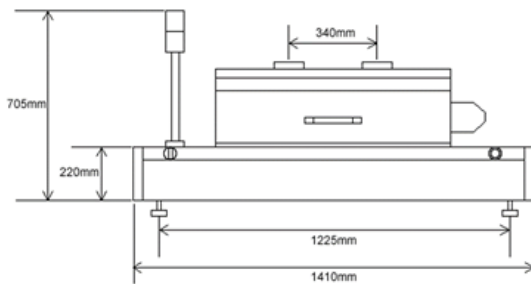
正视图
